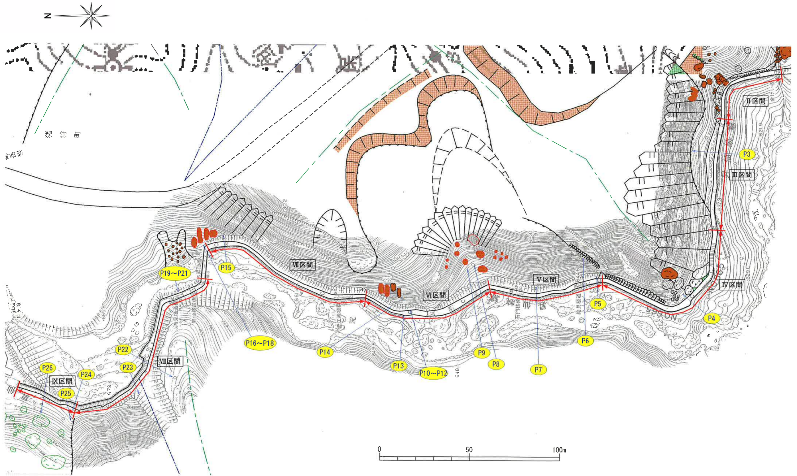
主要危険箇所位置図
